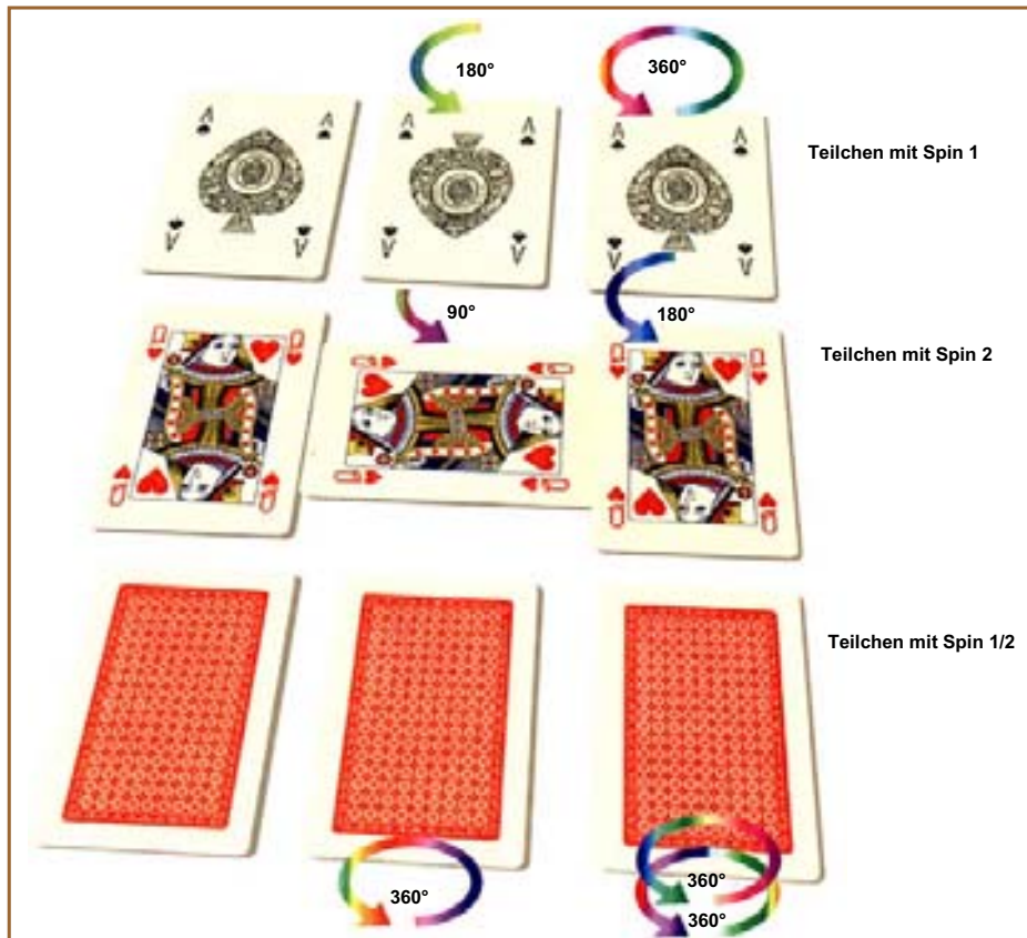
(Abb. 2.12) TEILCHENSPIN Alle Teilchen haben eine Eigenschaft, den Spin, von dem es abhängt, wie Teilchen unter verschiedenen Blickwinkeln aussehen. Das läßt sich an einem Kartenspiel anschaulich machen. Betrachten wir zunächst das Pik-As. Gleich sieht es nur nach einer vollständigen Umdrehung von 360 Grad aus. Daher sagt man, es habe Spin 1. Dagegen besitzt die Herzdame zwei Köpfe und sieht schon nach einer halben Umdrehung von 180 Grad gleich aus. Bei ihr spricht man von Spin 2. Entsprechend kann man sich Objekte mit Spin 3 oder mehr vorstellen, die schon bei kleineren Bruchteilen einer Umdrehung gleich aussehen. Je höher der Spin, desto kleiner der Bruchteil einer vollständigen Umdrehung, der erforderlich ist, um das Teilchen gleich aussehen zu lassen. Bemerkenswert - und nicht anhand von Alltagsgegenständen darstellbar - ist der Umstand, daß es auch Teilchen gibt, die sich selbst erst wieder gleichen, wenn sie zwei vollständige Umdrehungen hinter sich haben. In diesen Fällen spricht man von Spin 1/2.
