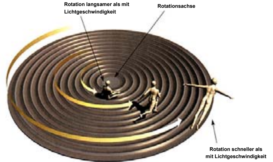
(Abb. 5.17) Im flachen Raum werden sich Regionen eines in starrer Rotation befindlichen Körpers fern von der Achse schneller als das Licht bewegen.
