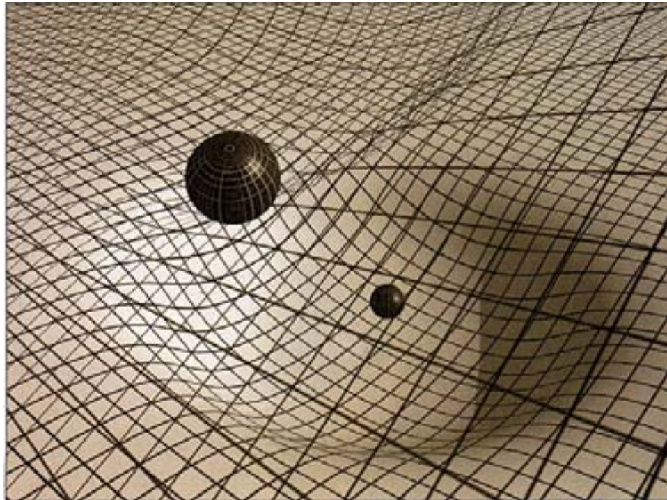
(Abb. 1.12) RAUMZEIT IST GEKRÜMMT Beschleunigung und Gravitation können nur äquivalent sein, wenn ein massereicher Körper die Raumzeit krümmt und dadurch die Bahnen von Objekten in seiner Nachbarschaft beeinflusst.
