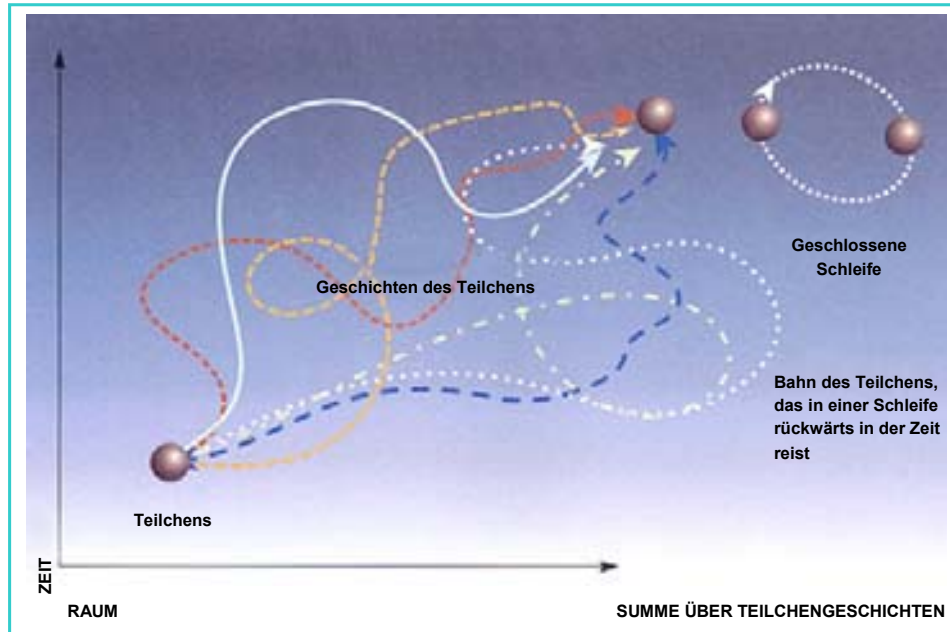
(Abb. 5.13) Die Feynmansche »Summe über Geschichten« muß auch Geschichten einschließen, in denen Teilchen in der Zeit zurückreisen, und sogar solche Geschichten, die geschlossene Schleifen in Zeit und Raum sind.
