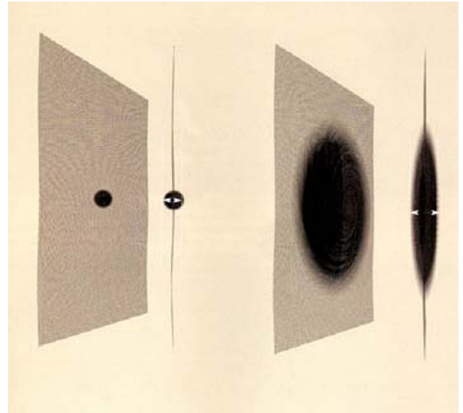
(Abb. 7.16) Ein Schwarzes Loch in unserer Welt auf der Bran würde sich in die Zusatzdimensionen ausdehnen. Wäre es klein, dann wäre es fast rund, doch ein großes Schwarzes Loch auf der Bran würde, bezieht man die Extradimensionen ein, wie ein abgeflachtes, pfannkuchenartiges Gebilde aussehen.
