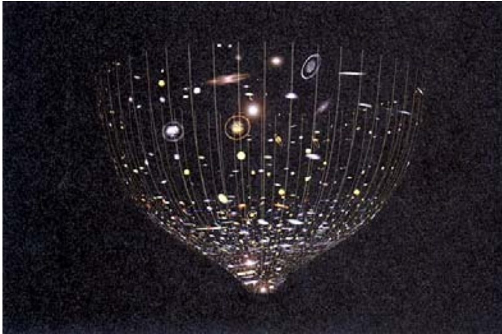
(Abb. 1.14) Beobachtungen von Galaxien lassen darauf schließen, daß das Universum expandiert: Die gegenseitige Entfernung nimmt für fast jedes Paar von Galaxien zu.
