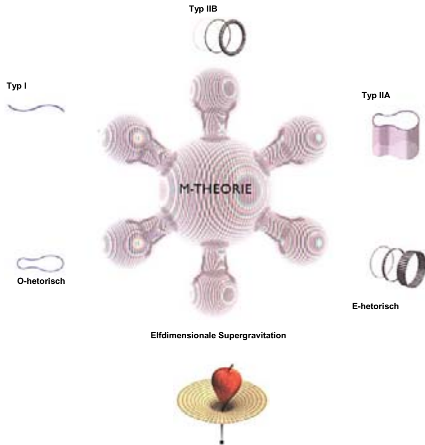
(Abb. 2.16) EIN VEREINHEITLICHTER THEORETISCHER RAHMEN?
