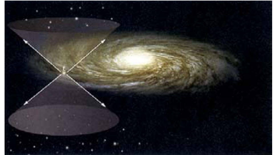
(Abb. 3.2) Unser Planet Erde (E) umkreist die Sonne in einer äußeren Region der Spiralgalaxie Milchstraße. Der Sternstaub in den Spiralarmen verwehrt uns den Blick in der Ebene der Galaxie, aber wir haben einen ungehinderten Blick zu beiden Seiten der Ebene.
