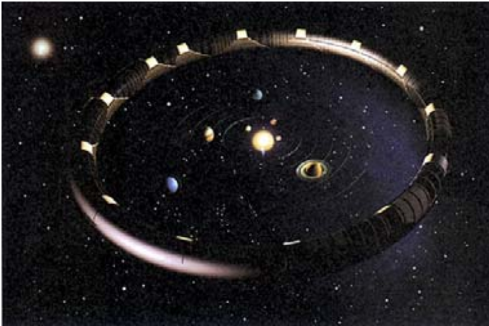
(Abb. 7.5) Ein Beschleuniger, der erforderlich ist, um Aufschluß über so kleine Abstände wie die Planck-Länge zu geben, wäre größer als der Durchmesser des Sonnensystems.
