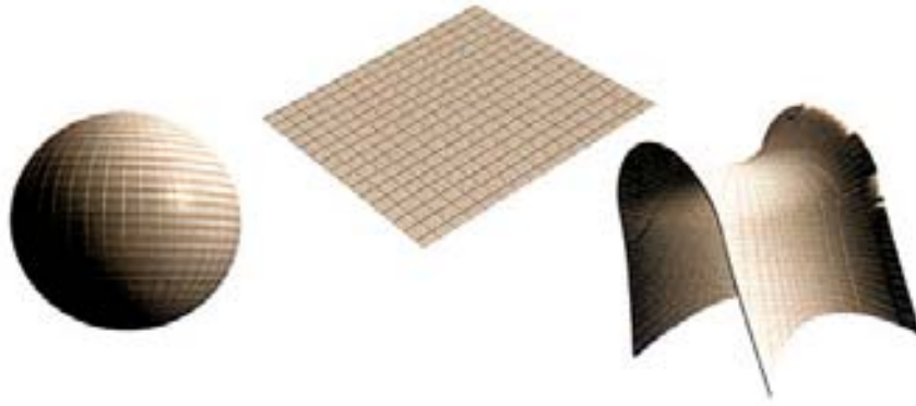
(Abb. 3.9) GESCHICHTEN DES UNIVERSUMS Wenn sich die Geschichten des Universums wie ein Sattel ins Unendliche erstrecken würden, stünde man vor der Schwierigkeit, die Randbedingungen im Unendlichen anzugeben. Wären alle Geschichten des
