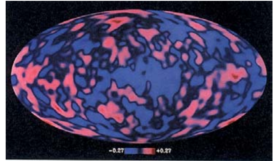
Die vollständige Himmelskarte, die das Mikrowellenradiometer DMR des Satelliten COBE geliefert hat, enthält Hinweise auf winzige Raumzeitkräuselungen.
