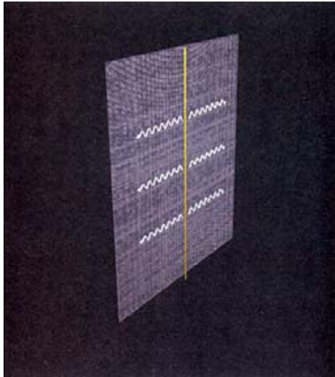
(Abb. 7.7) BRANWELTEN Die elektrischen Kräfte wären auf die Bran beschränkt und nähmen in dem Maße ab, das erforderlich wäre, um Elektronen mit stabilen Orbits um Atomkerne auszustatten.
