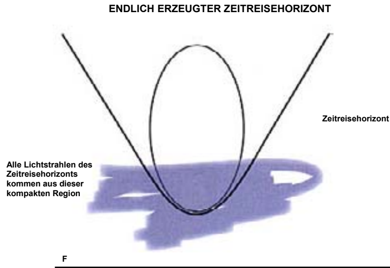
(Abb. 5.8) Selbst die fortgeschrittenste Zivilisation könnte die Raumzeit lediglich in einem endlichen Gebiet krümmen. Der Zeitreisehorizont, der Rand derjenigen Raumzeitregion, in der es möglich ist, in die eigene Vergangenheit zu reisen, wird durch Lichtstrahlen gebildet, die in einer endlichen Region ihren Anfang nehmen.
