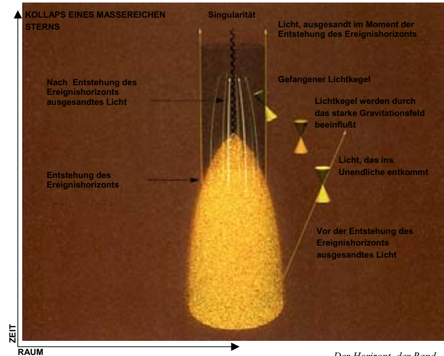
Der Horizont, der Rand des Schwarzen Lochs, wird von Lichtstrahlen gebildet, die es gerade nicht mehr schaffen, dem Schwarzen Loch zu entkommen, sondern gezwungen werden, ewig auf derselben Raumfläche zu verharrten.
