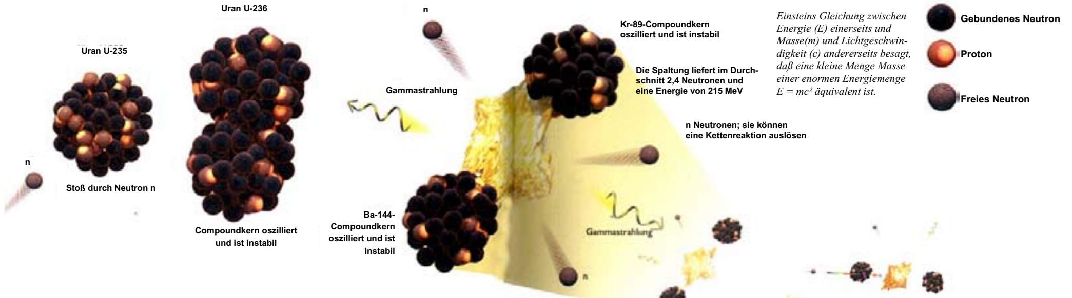
(Abb. 1.8) NUKLEARE BINDUNGSENERGIE Kerne bestehen aus Protonen und Neutronen. Doch die Masse eines Kerns ist stets geringer als die Summe der individuellen Massen seiner Protonen und Neutronen. Diese Massendifferenz \Delta m geht auf die Bindungsenergie zurück, die den Kern zusammenhält; gemäß Einsteins berühmter Formel ist die Bindungsenergie gleich \Delta mc^2 . Sie kann für unterschiedliche Kerne unterschiedlich groß sein; die Bindungsenergien der am Spaltungsprozeß beteiligten Kerne sind gerade dergestalt, daß die Masse des Einzelkerns vor der Spaltung größer ist als die Summe der Massen der Teilkerne danach. Durch die Entfesselung dieser Massendifferenz in Form von Energie wird die verheerende Explosivkraft der Kernwaffen erzeugt.
