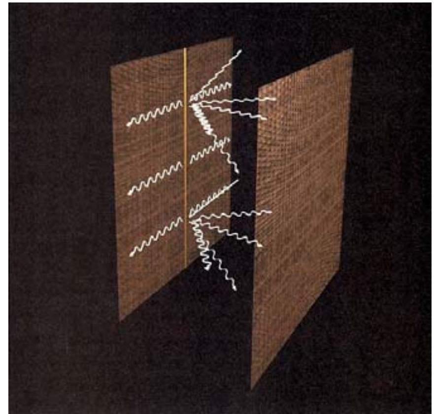
(Abb. 7.10) Eine zweite Bran in der Nähe unserer Branwelt würde die Gravitation daran hindern, sich weit in die zusätzlichen Dimensionen auszubreiten, und dazu führen, daß die Gravitation bei Entfernungen, die größer als der Branabstand sind, in einem Maße abfiel, wie es bei vier Dimensionen zu erwarten wäre.
