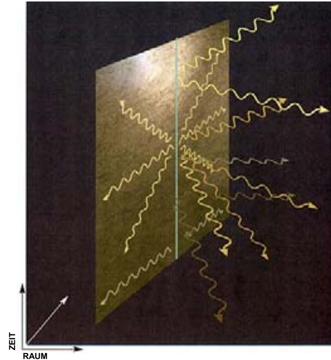
(Abb. 7.8) Die Gravitation würde nicht nur entlang der Bran wirken, sondern sich auch in die zusätzlichen Dimensionen ausbreiten und daher mit wachsender Entfernung rascher abnehmen als in vier Dimensionen.
