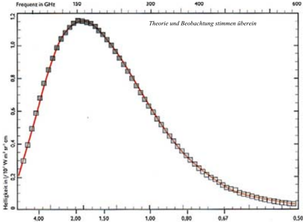
(Abb. 2.6) DAS SPEKTRUM DER KOSMISCHEN HINTERGRUNDSTRAHLUNG Das Spektrum - die Verteilung der Strahlungsleistung auf die verschiedenen Frequenzen - der kosmischen Hintergrundstrahlung ist typisch für das Strahlungsspektrum eines heißen Körpers. Um ein Wärmegleichgewicht zu erreichen, müssen Strahlung und Materie viele Male aneinander gestreut haben. Daraus läßt sich auf eine Materiedichte in der Vergangenheit schließen, die ausreichte, um unseren Vergangenheitslichtkegel nach innen zu biegen.
