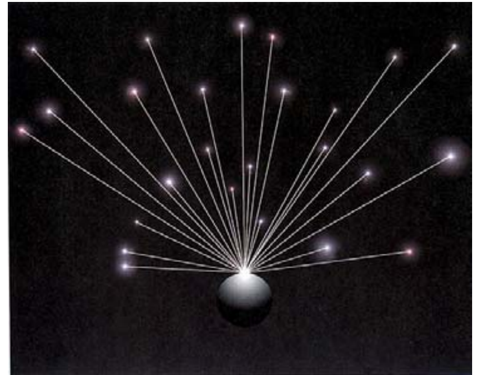
(Abb. 3.4) Wäre das Universum statisch und in jeder Richtung unendlich, würde jede Sichtlinie an einem Stern enden, so daß der Nachthimmel hell wie die Oberfläche der Sonne wäre.
