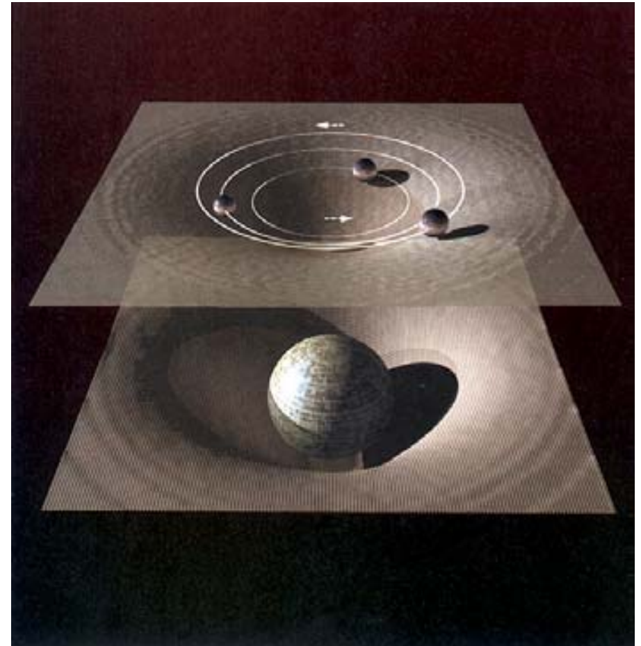
(Abb. 7.12) Im Branwelt-Szenario könnten Planeten eine dunkle Masse auf einer Schattenbran umkreisen, weil sich die Gravitationskraft in die zusätzlichen Dimensionen ausbreitet.
