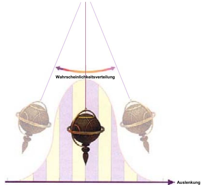
(Abb. 2.10) PENDEL MIT WAHRSCHEINLICHKEITSVERTEILUNG Nach der Quantentheorie muß ein Pendel selbst in seinem niedrigsten Energiezustand ein Minimum an Fluktuationen aufweisen. Seine Position ist durch eine Wahrscheinlichkeitsverteilung gegeben: Im Grundzustand ist die wahrscheinlichste Position eine Ausrichtung, die direkt nach unten zeigt, aber es besteht auch eine gewisse Wahrscheinlichkeit, das Pendel in einem kleinen Winkel zur Senkrechten anzutreffen.
