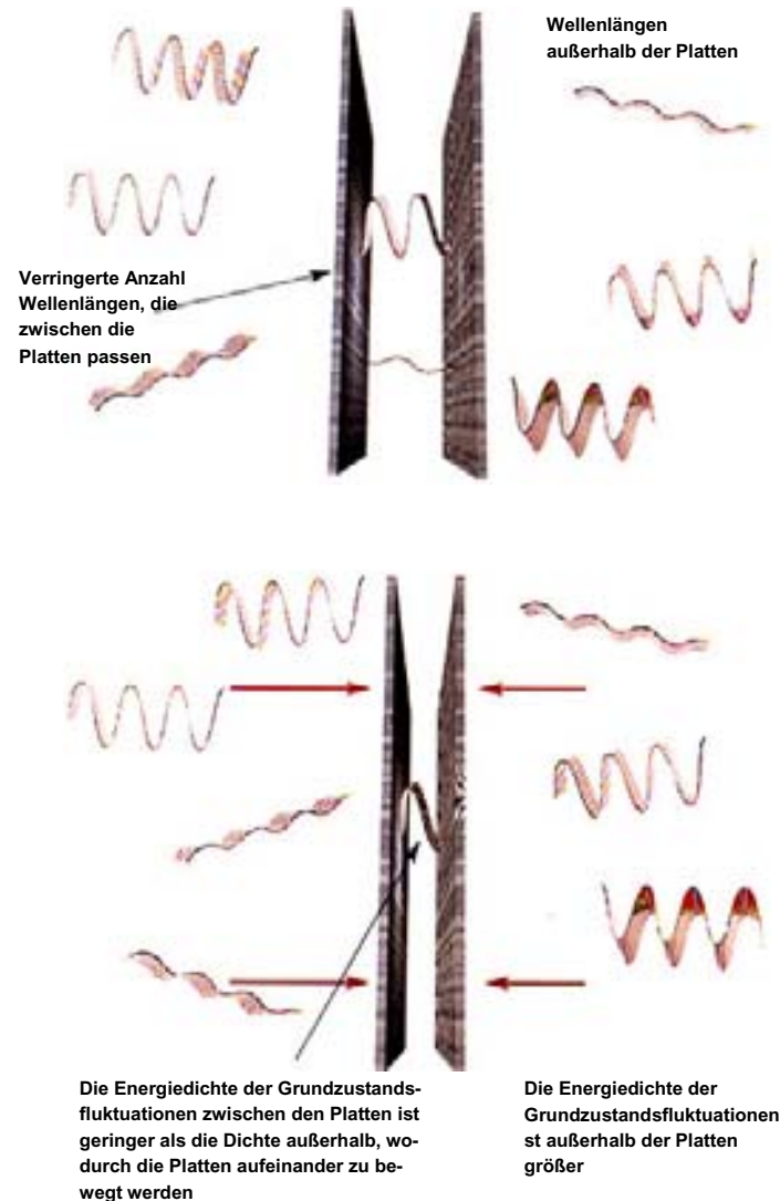
(Abb. 2.11) DER CASIMIR-EFFEKT Die Existenz von Grundzustandsfluktuationen ist durch den experimentellen Nachweis des Casimir-Effekts bestätigt worden, einer winzigen Kraft, die zwischen parallelen, elektrisch neutralen Metallplatten wirkt.
