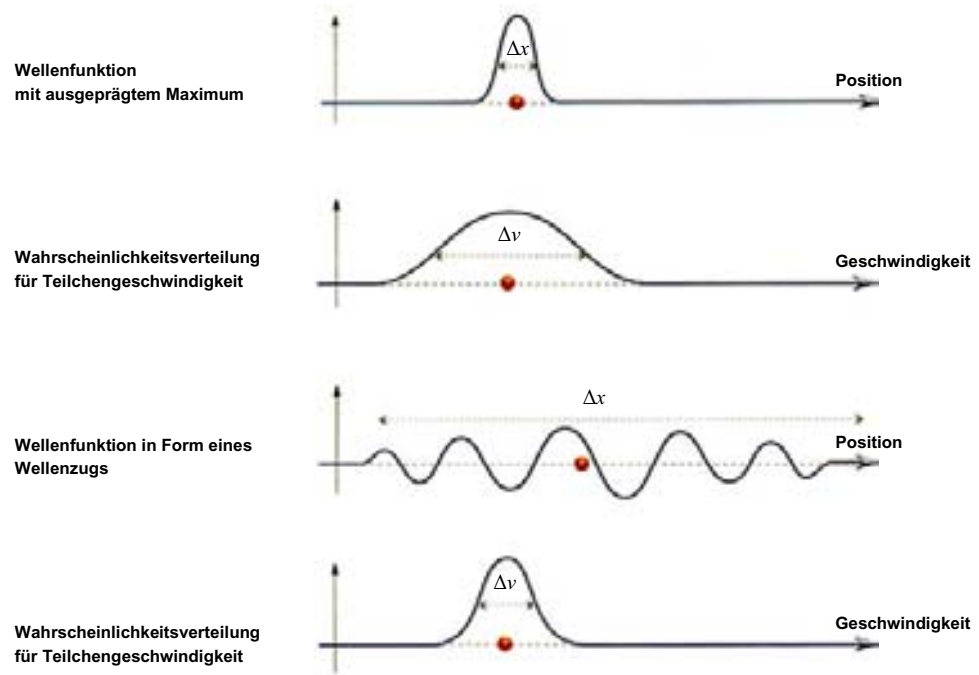
(Abb. 4.4) Die Wahrscheinlichkeit, das Teilchen an einem gegebenen Ort und mit einer gegebenen Geschwindigkeit anzutreffen, wird durch seine Wellenfunktion bestimmt, und zwar so, daß \Delta x und \Delta v der Unschärferelation gehorchen.
