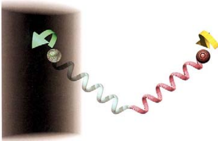
(Abb. 4.21) Ein virtuelles Teilchenpaar hat eine Wellenfunktion, die vorhersagt, daß die beiden Teilchen entgegengesetzte Spins haben. Doch wenn ein Teilchen in das Schwarze Loch fällt, läßt sich der Spin des verbleibenden Teilchens nicht mehr mit Gewißheit vorhersagen.
