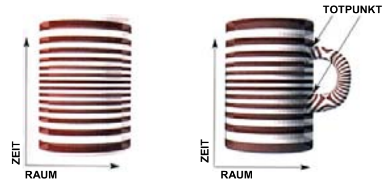
(Abb. 4.7) DIE ZEIT STEHT STILL Ein Zeitmaß hätte notwendigerweise dort Totpunkte, wo der Griff am Hauptzylinder ansetzt: Punkte, an denen die Zeit still stünde. An diesen Punkten nähme die Zeit in keiner Richtung zu. Daher könnte man mit der Schrödinger-Gleichung nicht vorherhersagen, wie die Wellenfunktion in Zukunft aussähe.
