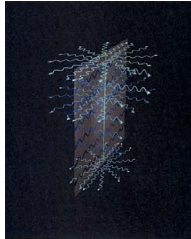
(Abb. 7.15) Im Randall-Sundrum-Modell können kurzwellige Gravitationswellen Energie von Quellen auf der Bran davontragen und scheinbare Verstöße gegen den Energieerhaltungssatz bewirken.
