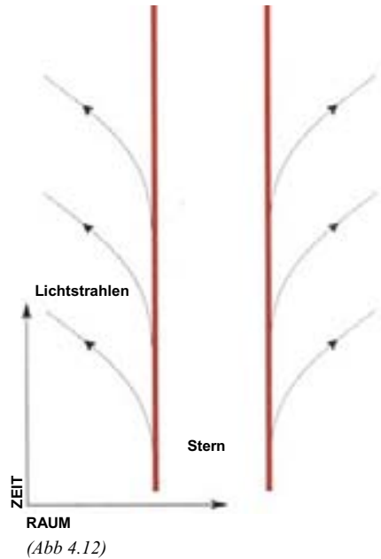
(Abb. 4.12) Die Raumzeit um einen stabilen Stern herum. Licht kann von der Oberfläche des Sterns (rote senkrechte Linien) in die Weiten des Alls entkommen. Weit von dem Stern entfernt verlaufen die Lichtbahnen im Winkel von 45 Grad zur Senkrechten; näher an der Sternoberfläche zwingt die Raumzeitkrümmung die Lichtbahnen, steiler zu verlaufen.
