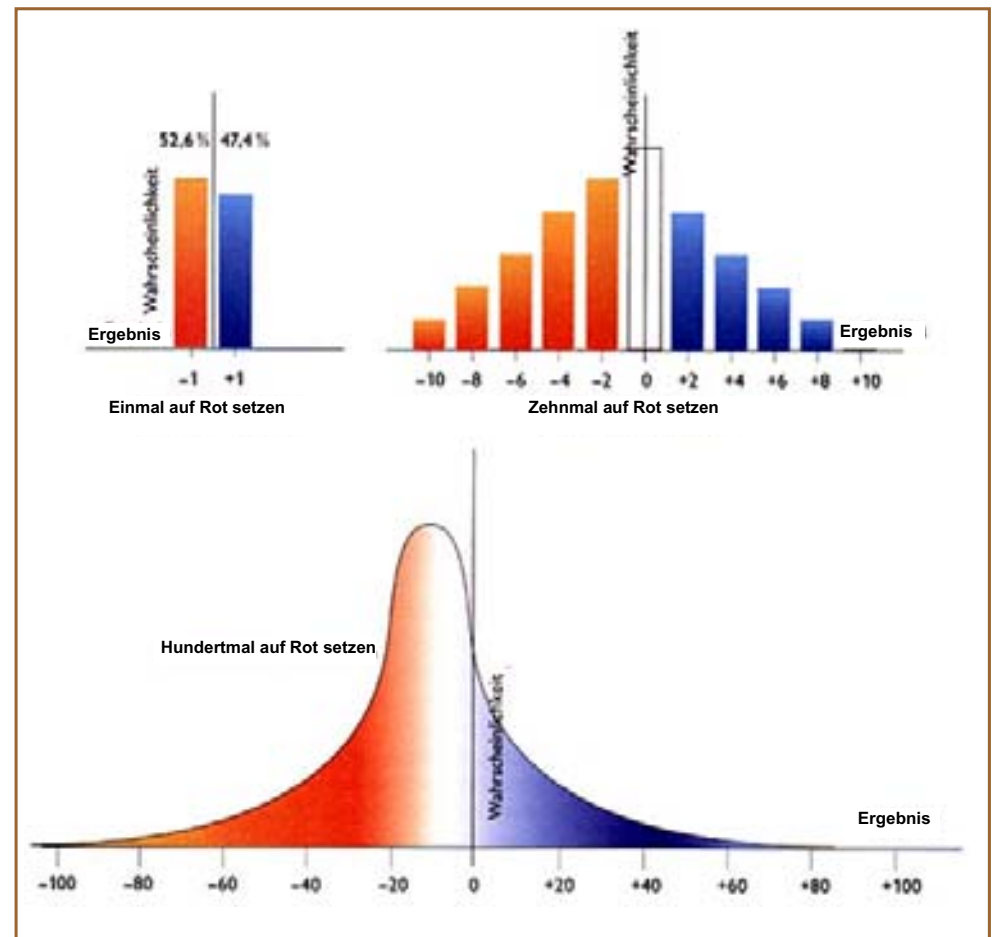
(Abb. 3.7 oben und Abb. 3.8 gegenüber) Wenn ein Roulettespieler bei einer großen Zahl von Spielen auf Rot setzt, kann man seinen Gewinn ziemlich genau vorhersagen, weil sich die Ergebnisse der einzelnen Spiele ausgleichen. Dagegen ist es unmöglich, das Ergebnis eines einzelnen Spiels vorherzusagen.
