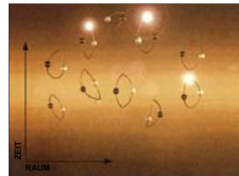
(Abb. 4.17) Oben: In der Nähe eines Schwarzen Lochs treten virtuelle Teilchen auf und vernichten sich wieder gegenseitig. Gelegentlich stürzt ein Partner des Paares in das Schwarze Loch, während seinem Zwilling die Flucht ins Freie gelingt. Von außen betrachtet scheint es, als emittiere das Schwarze Loch die entweichenden Teilchen.
