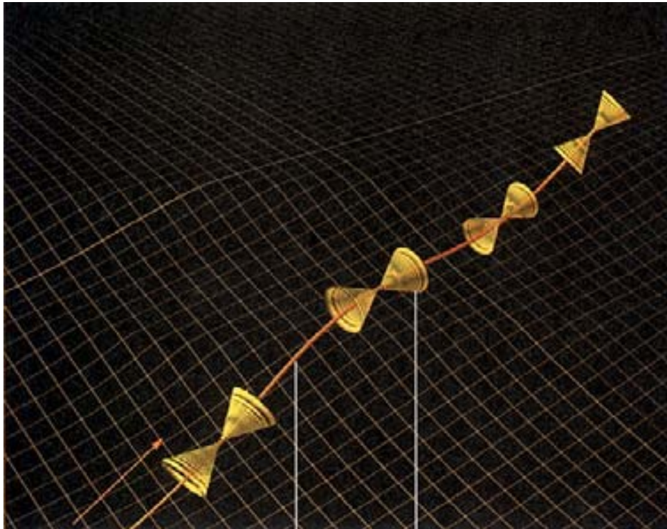
(Abb. 2.19) In der reellen Raumzeit der klassischen allgemeinen Relativitätstheorie unterscheidet sich die Zeit von den Raumrichtungen dadurch, daß sie entlang der Geschichte eines Beobachters nur zunehmen kann, anders als die Raumrichtungen, deren Koordinatenwerte entlang dieser Geschichte zu- oder abnehmen können.
