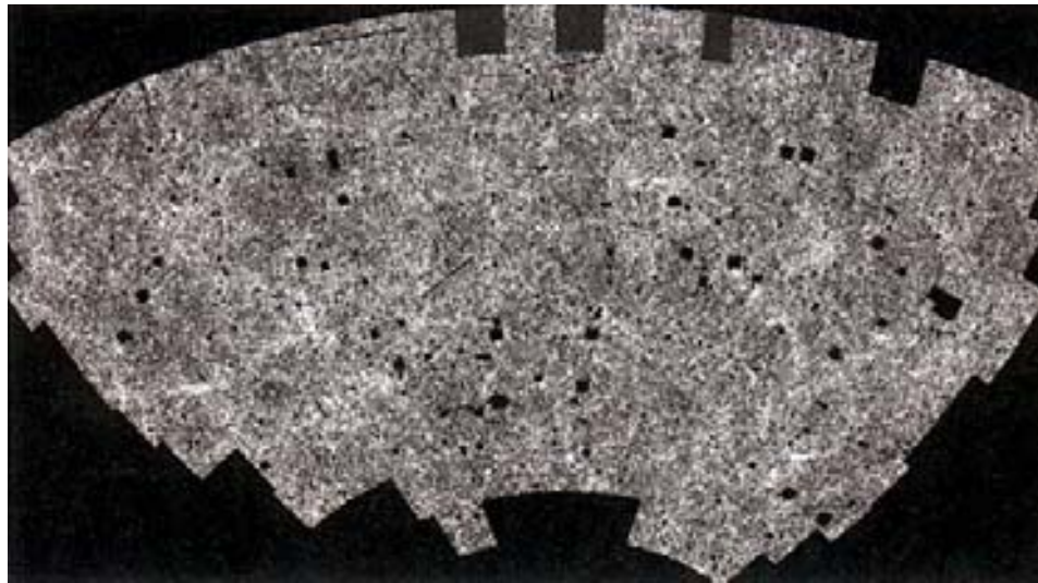
(Abb. 3.1) Wenn wir tief ins Universum hineinschauen, erblicken wir Milliarden und Abermilliarden von Galaxien. Galaxien können unterschiedliche Formen und Größen haben; sie können beispielsweise elliptisch sein oder spiralförmig wie unsere Heimatgalaxie, die Milchstraße.
