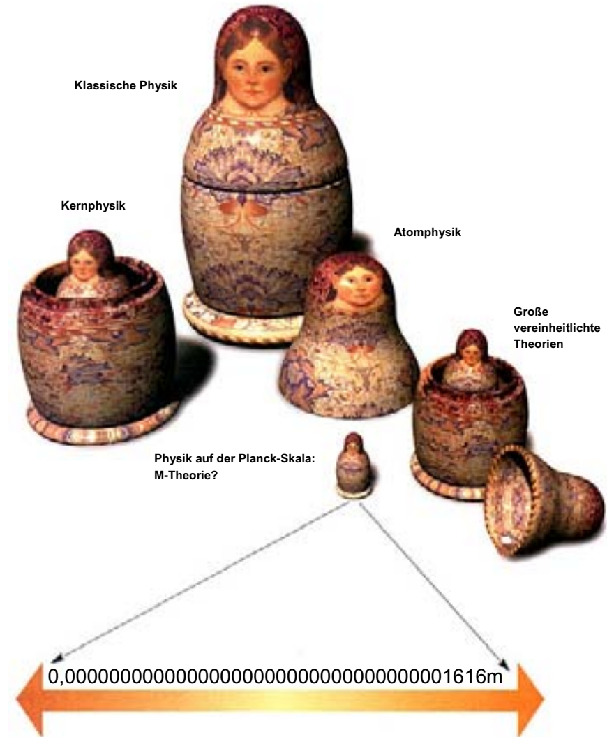
(Abb. 7.4) Jede Puppe steht für ein theoretisches Naturverständnis bis hinab zu einer bestimmten Längenskala. Jede enthält eine kleinere Puppe, das heißt, eine Theorie, die die Natur auf noch kleineren Skalen beschreibt. Aber es gibt eine kleinste fundamentale Länge in der Physik, die Planck-Länge, eine Skala, auf der die Natur möglicherweise durch die M-Theorie beschrieben wird.
