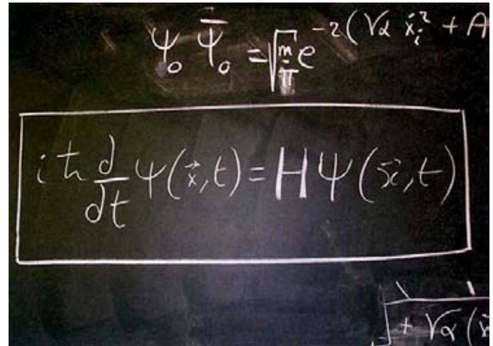
(Abb. 4.5) DIE SCHRÖDINGER-GLEICHUNG Wie sich die Wellenfunktion \Psi entwickelt, wird durch den Hamilton-Operator H bestimmt, der mit der Energie des betreffenden physikalischen Systems zusammenhängt.
