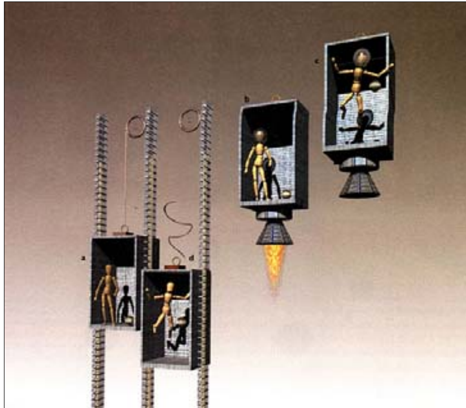
(Abb. 1.9) Ein Beobachter in einer Kiste kann nicht entscheiden, ob er sich in einem auf der Erde ruhenden Fahrstuhl befindet (a) oder von einer Rakete im freien Raum beschleunigt wird (b). Wenn der Raketenantrieb abgeschaltet wird (c), hat der Beobachter das gleiche Empfinden wie in einem Fahrstuhl, der sich in freiem Fall zum Boden des Schachts befindet (d).
