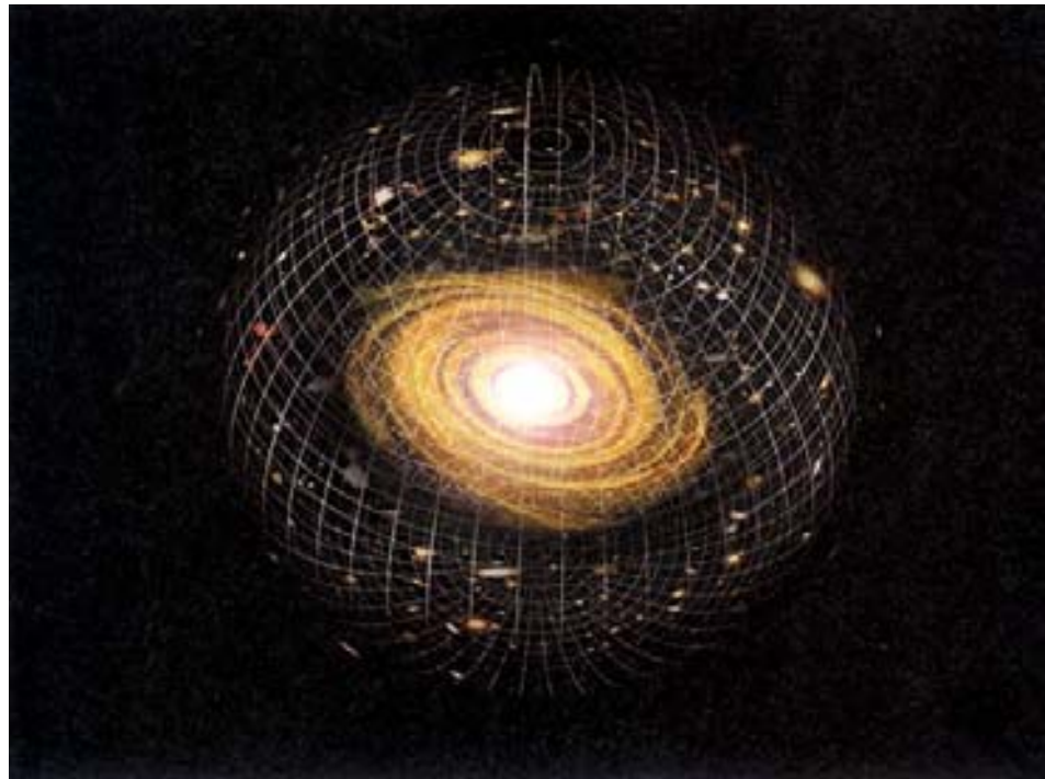
(Abb. 3.18, oben) Ein mögliches Ende des Universums ist der Große Endkollaps, in dessen Verlauf das All zu einem Gebilde extremer Dichte zusammenstürzen würde.
