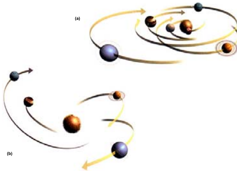
Abb. 7.9) Eine raschere Abnahme der Gravitationskraft bei größeren Abständen würde bedeuten, daß Planetenbahnen instabil wären. Die Planeten stürzten entweder in die Sonne (a) oder entfernten sich ganz aus ihrer Anziehung (b).
