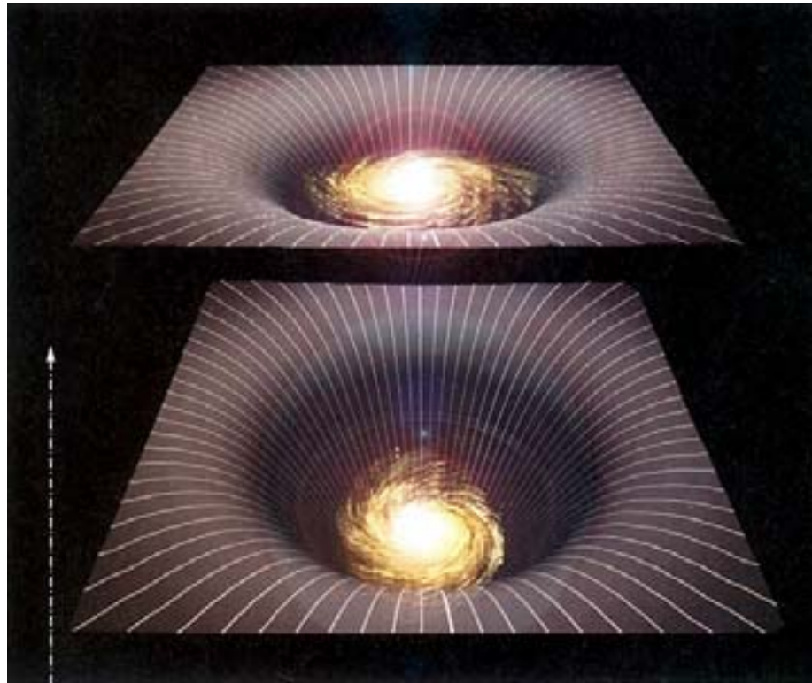
Das Niemandsland der Zusatzdimension zwischen den Branen
