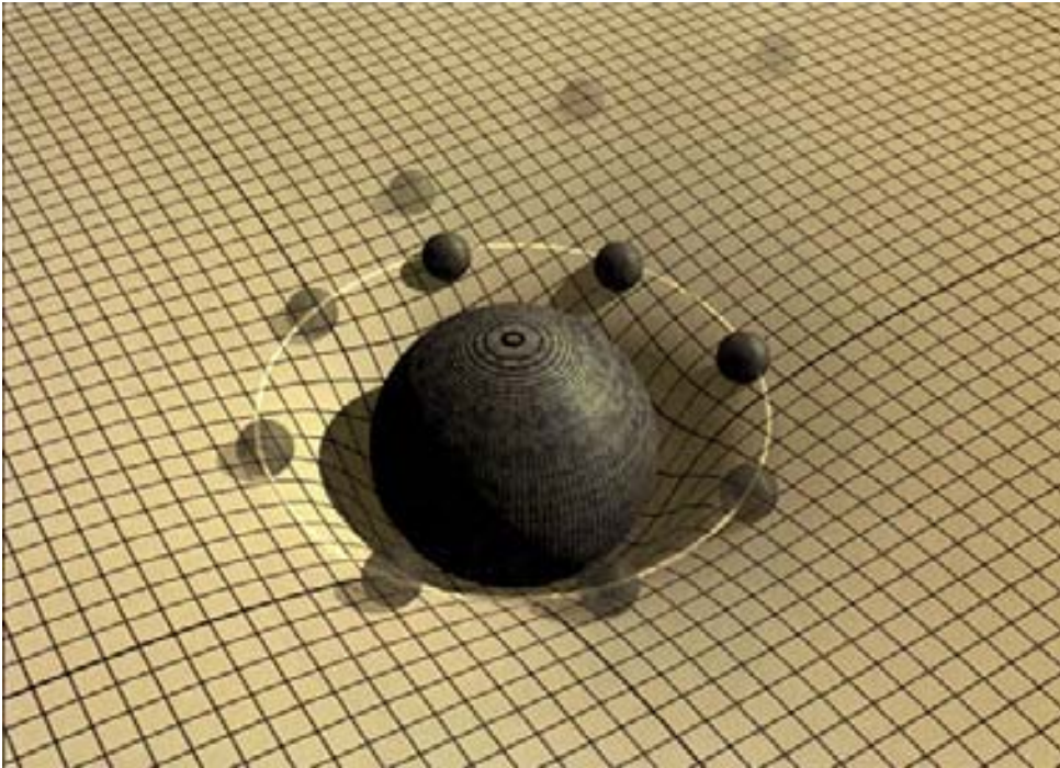
(Abb. 2.4) DIE GUMMITUCHANALOGIE Die große Kugel in der Mitte stellt einen massereichen Körper dar, beispielsweise einen Stern. Sein Gewicht krümmt das Tuch in seiner Umgebung. Die kleinen Kugeln, die auf dem Tuch rollen, werden von der Krümmung abgelenkt und umrunden die große Kugel, ähnlich wie Planeten im Gravitationsfeld eines Sterns diesen umkreisen.
