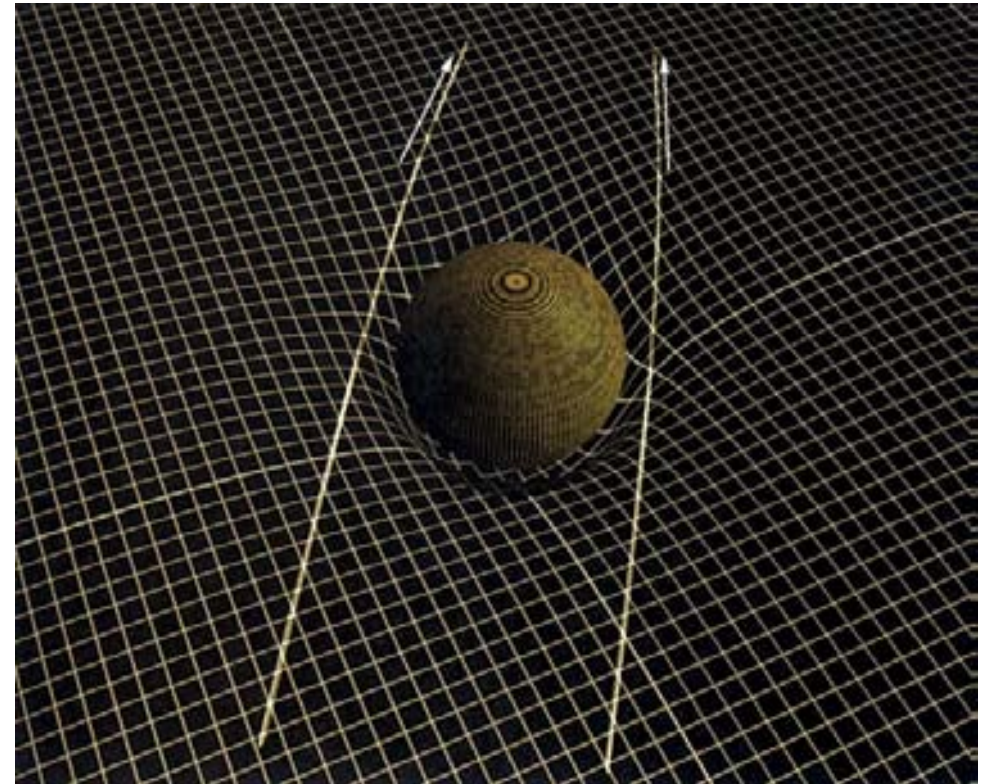
(Abb. 2.7) KRÜMMUNG DER RAUMZEIT Weil die Gravitation eine anziehende Kraft ist, bewirkt Materie immer eine Krümmung der Raumzeit, durch die Lichtstrahlen aufeinander zu gelenkt werden.
