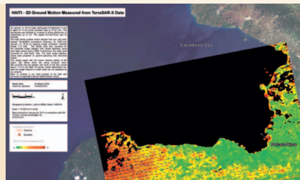
Der deutsche Erdbeobachtungssatellit TerraSAR-X lieferte nach dem Erdbeben von Haiti Anfang 2010 Daten zur Erdkrustenbewegung: grün bedeutet kaum Verschiebung, rot zwei Meter Bewegung.
