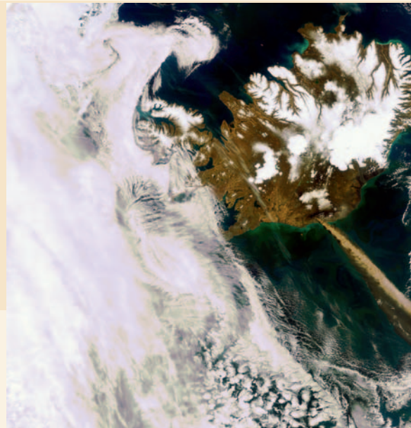
Die dichte Aschewolke des isländischen Vulkans Eyjafjallajökull aus Sicht des europäischen Erdbeobachtungssatelliten ENVISAT im April 2010
