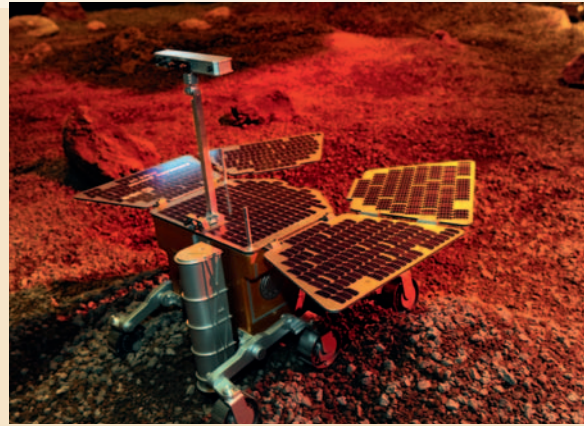
DLR-Studie für einen Marsrover
